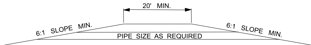
SECTION A-A
